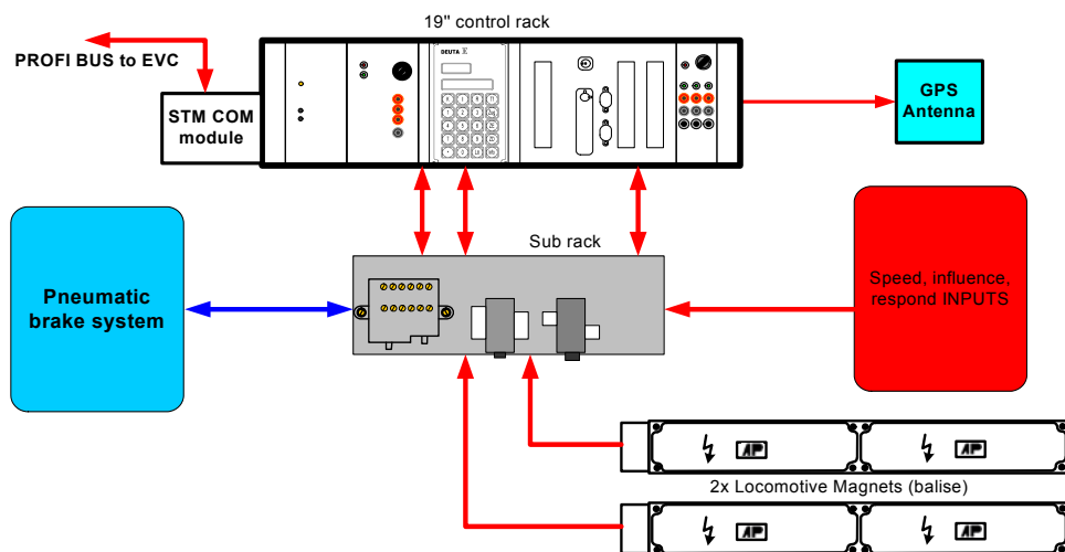
Slika 1. Blok dijagram APAS0408 sustava
